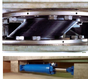
積層ゴムの変形
